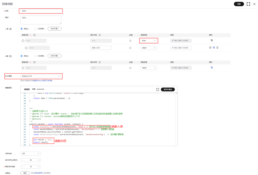
图 3-2 创建函数
